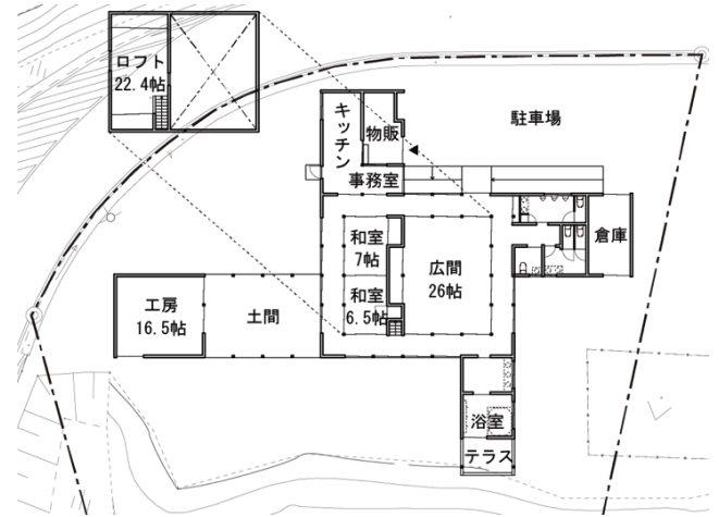
図 1 波板地域交流センターの平面図
